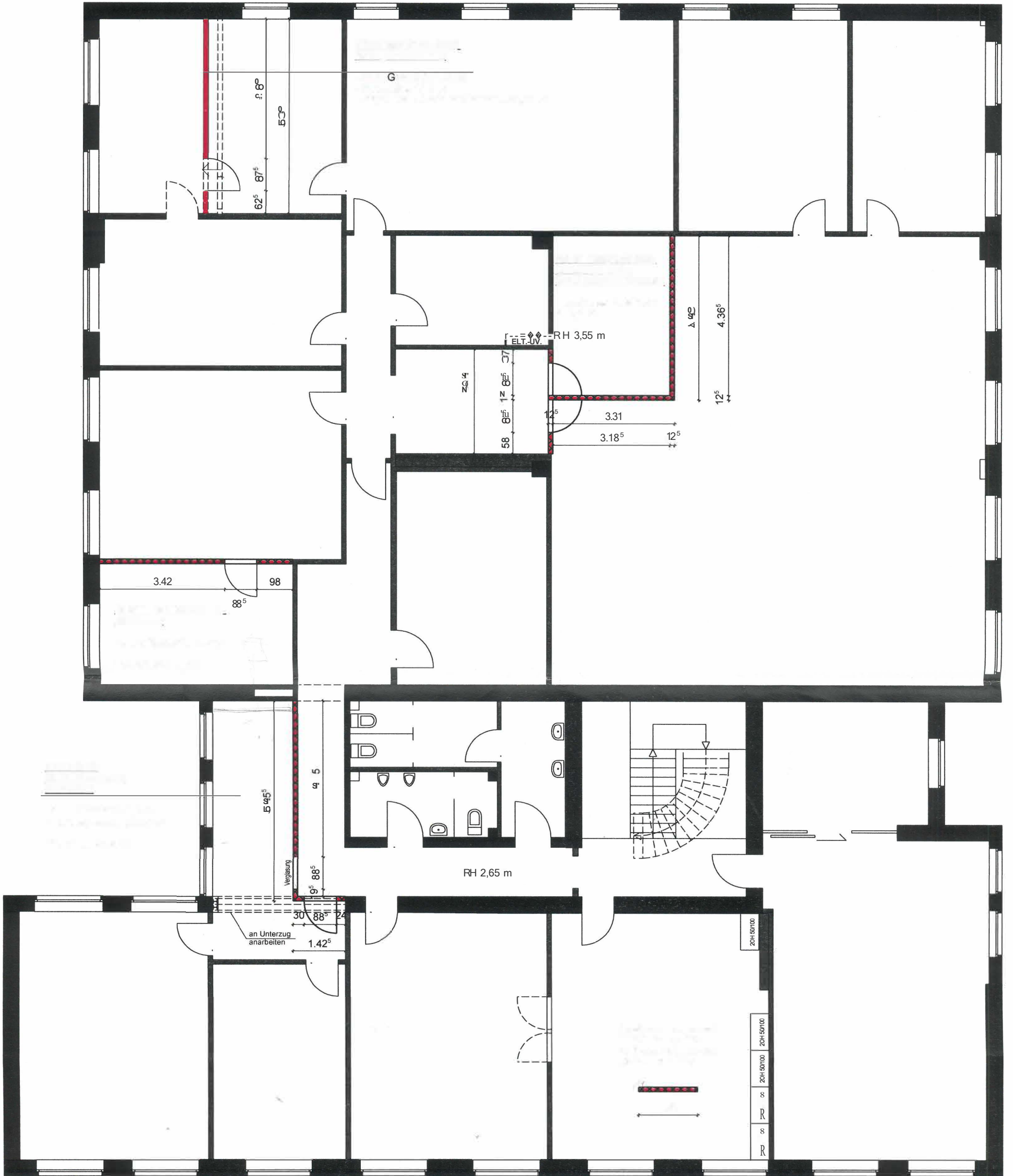
GRUNDRISS 1. OG M 1:100
